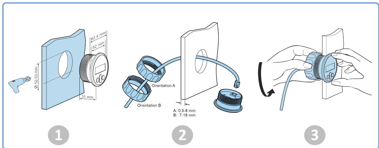
Monteringsmetod A.
